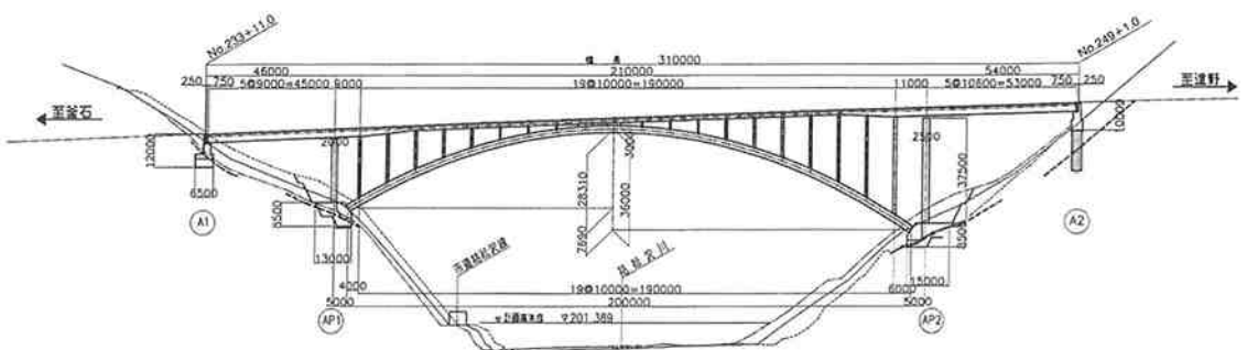
図-2 正面図
