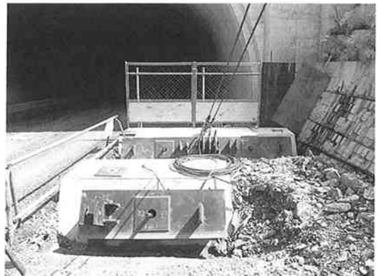
写真-4 A1ケーブルクレーンアンカー
