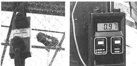
写真-10 テンションメーター及び遠隔モニター
