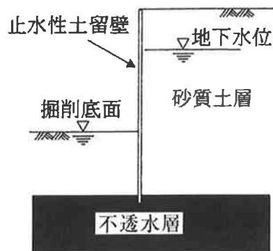
(a) 根入れ長増加および地盤改良
