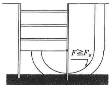
(a) 根入れ長増加および地盤改良
