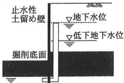
(b) 揚水による方法
