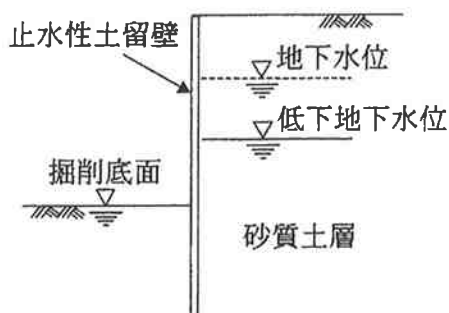
(b) 背面地盤地下水位低下 図-2 ボーリングに対する対策
