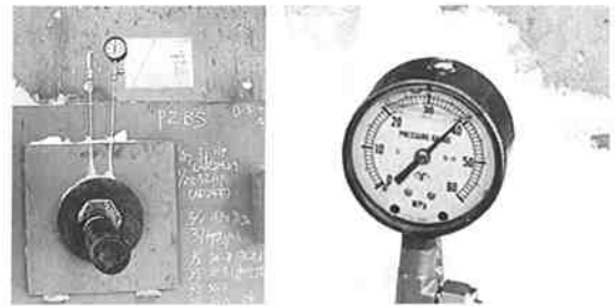
写真-12 ロードセルとプレッシャーゲイジ
