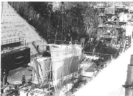
写真-6 ジョイント部養生状況
