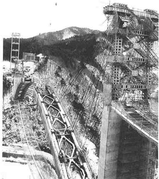
写真-1 厳冬の斜吊架設（平成18年2月）
