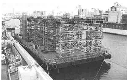
写真-2 ベント設置状況
