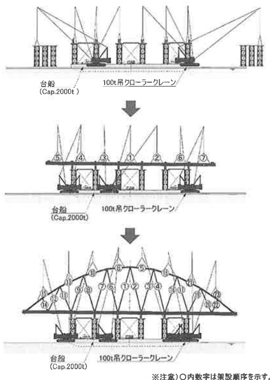
図-2 架設ステップ
