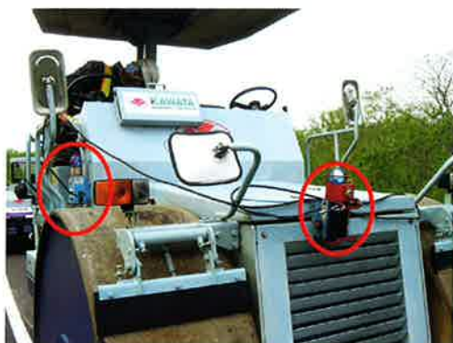
写真ー3 センサー取付位置
