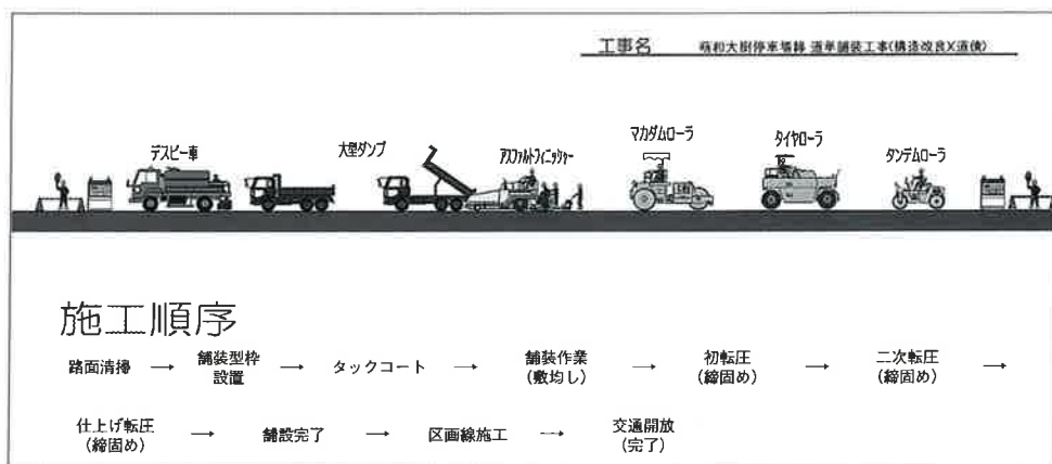
図ー1 表層・基礎工施工図
